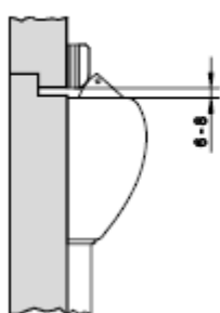
Плоский ограничитель двери
