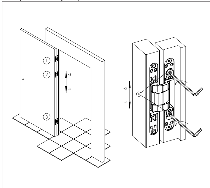
Рисунок 4 — Вертикальная регулировка.
