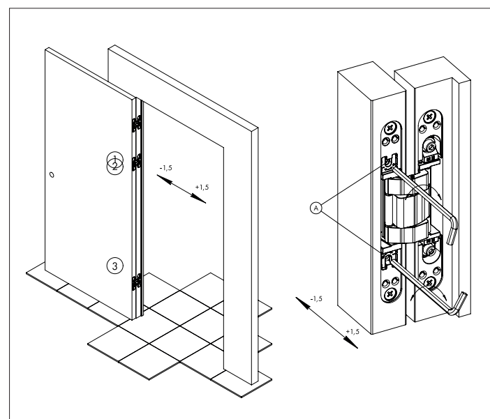
Рисунок 3 — Горизонтальная регулировка.
