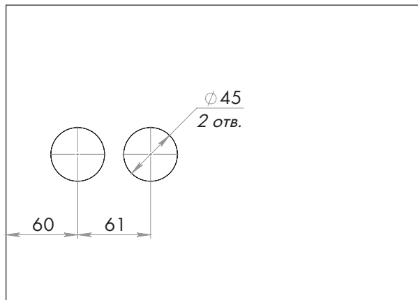
Эскиз подготовки стекла.
