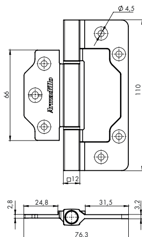
Рисунок 1 – Габаритные размеры петель.
