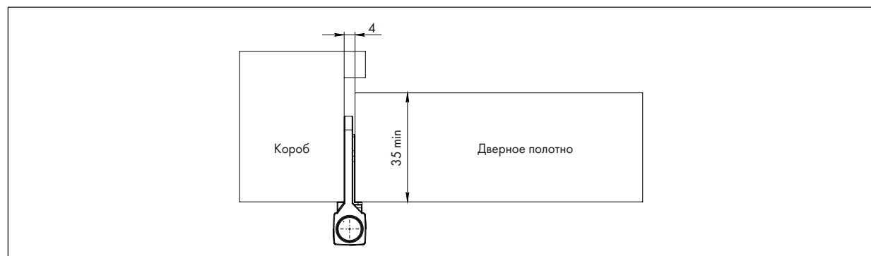
Рисунок 3 – Схема расположения петель.
