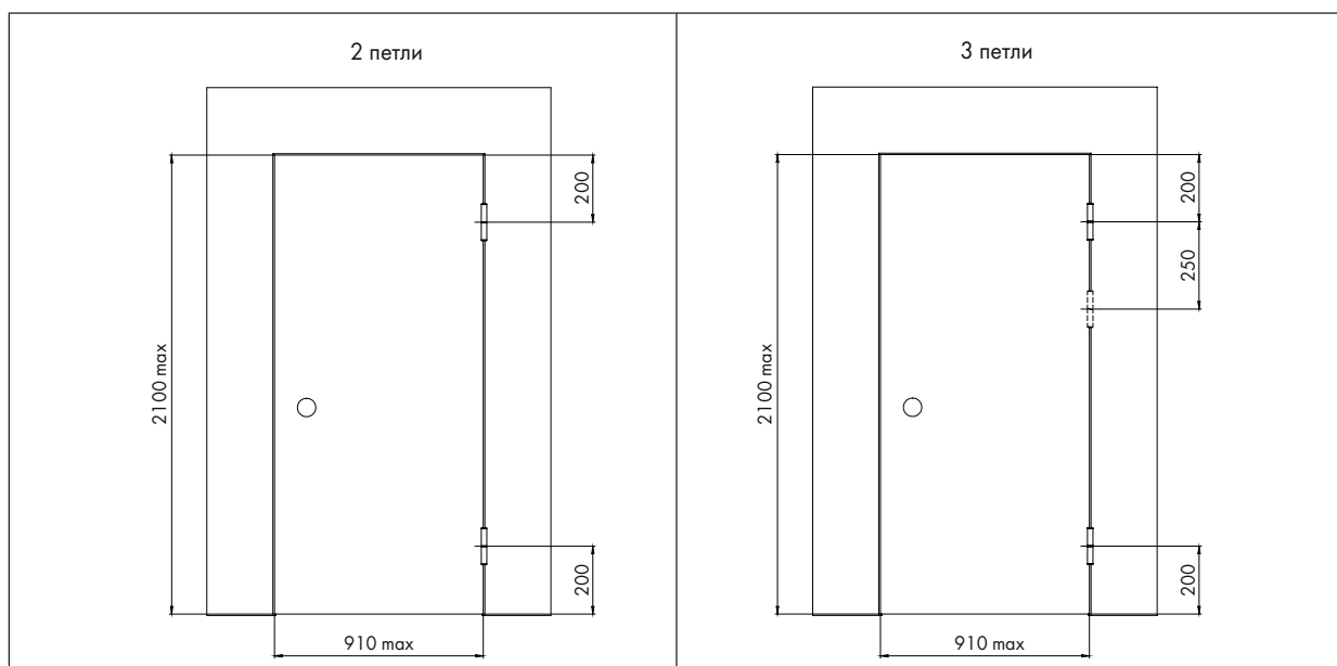
Рисунок 2 – Схема расположения петель (2 петли/3петли).
