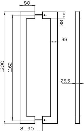
PULL.PH38/1200.26 INOX
