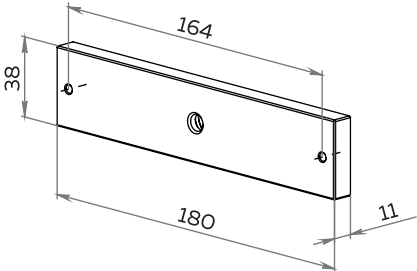
поз. 4 – Пластина
