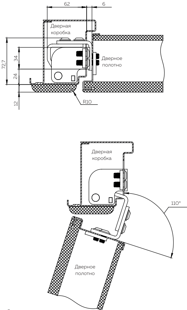
Рисунок 2 Расположение петель
