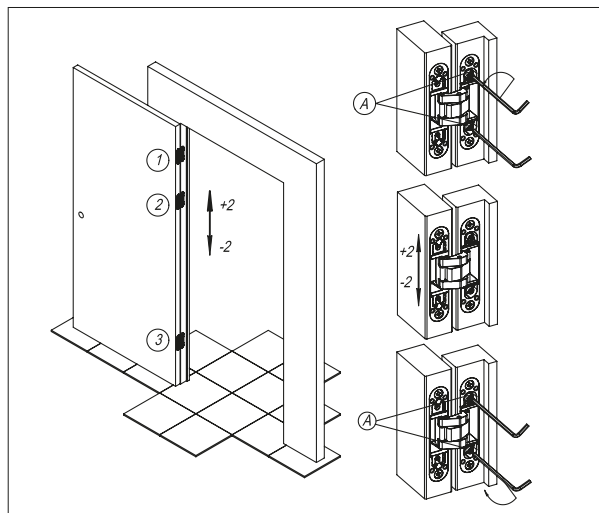
Рисунок 3 — Вертикальная регулировка.
