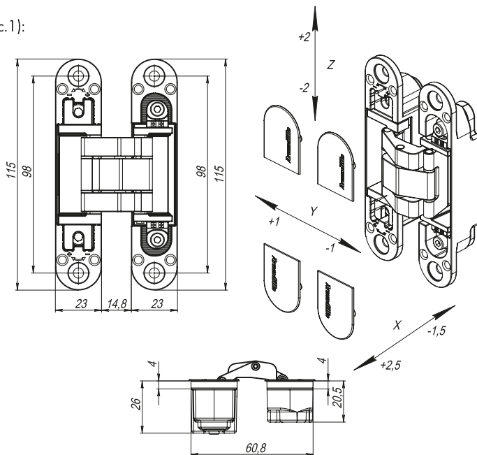
Рисунок 1 — Габаритные размеры петель.
