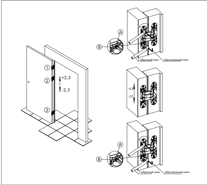
Рисунок 6 — Вертикальная регулировка.
