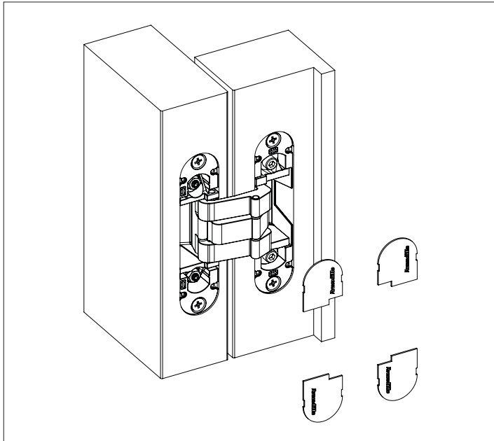
Рисунок 8 — Установка декоративных накладок.
