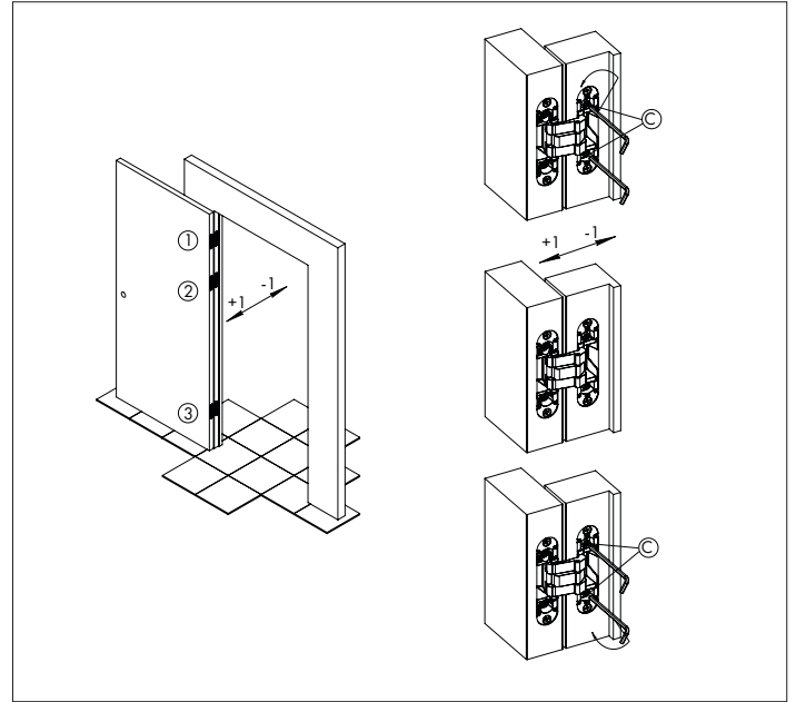
Рисунок 7 — Регулировка по глубине.
